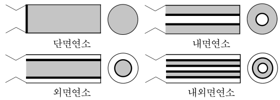
— 그레이의 연소면 그레이 <그림 1> 단면 형상에 따른 그레이의 연소 방식
